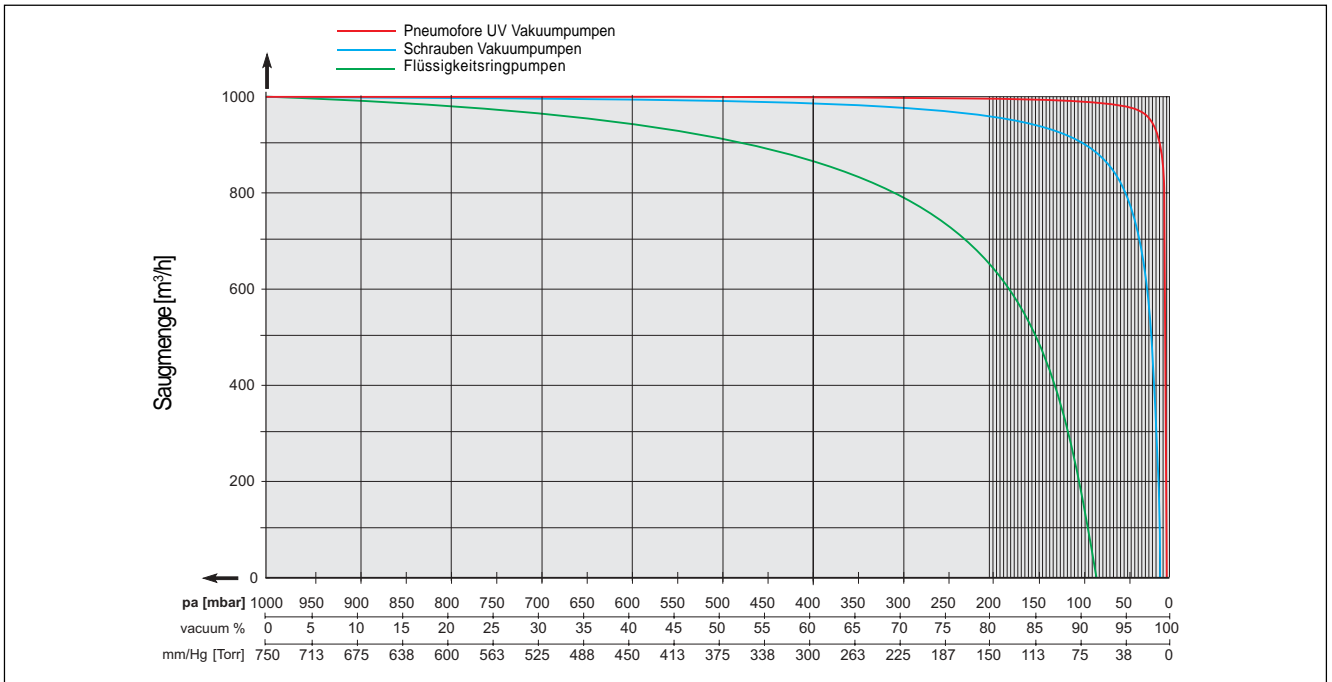
Abb. 2 - Vergleich verschiedener Bauarten – Verlauf des Ansaugvolumens bei Veränderung des Vakuums
