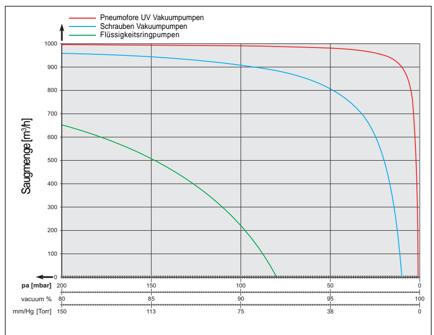
Abb. 3 - Vergrößerung des schraffierten Arbeitsgebietes unterhalb 200 mbar
