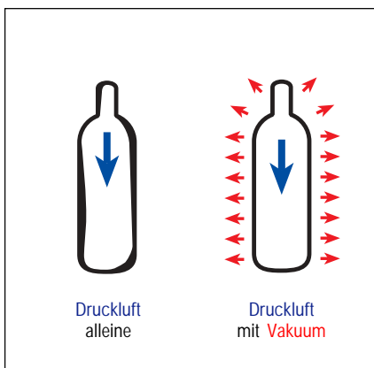
Abb. 4 - Die Vorteile des Vakuums bei der Herstellung von Glasflaschen
